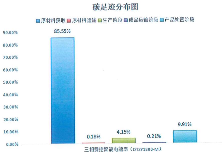
图 5.2-2 三相费控智能电能表（DTZY1800-M） 生命周期阶段碳排放分布图
