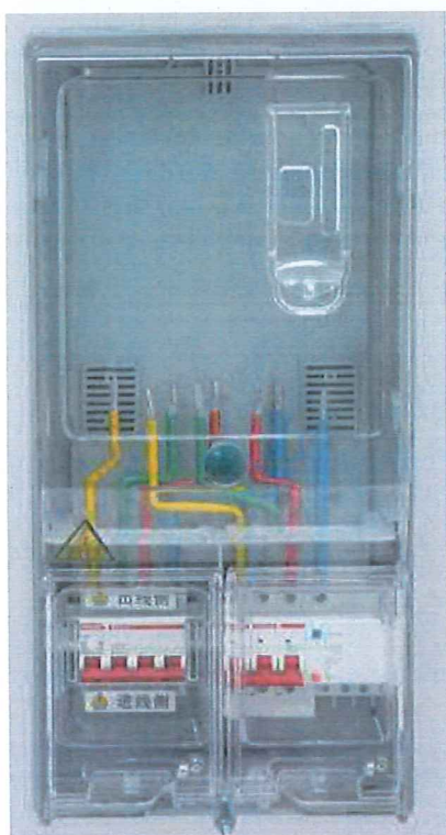
电 能 计 量 箱
