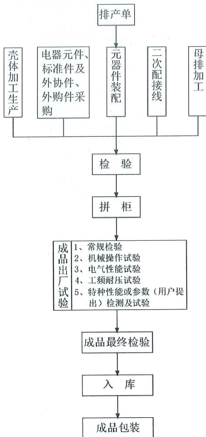
落地计量产品工艺流程图
