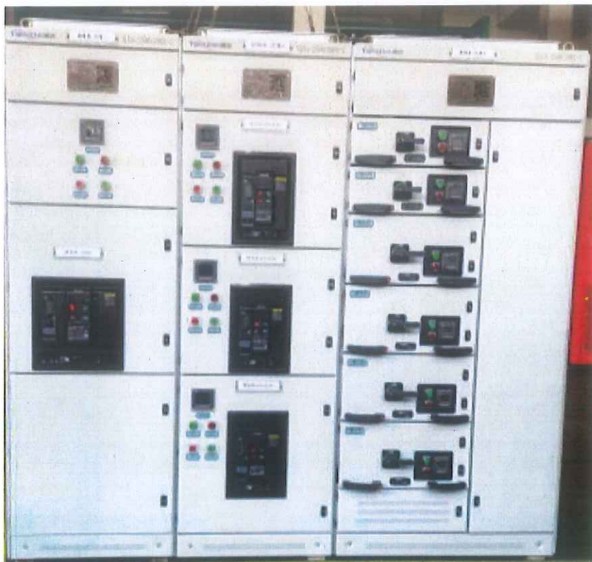
低压成套设备
