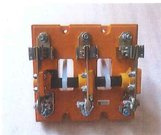
低压刀开关
