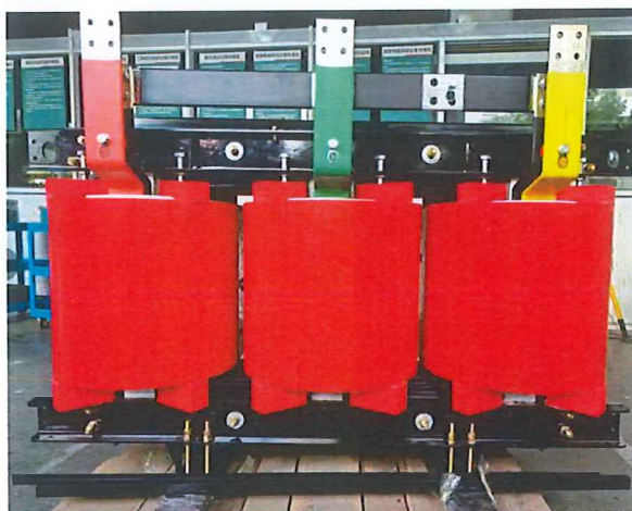
配电变压器（干式）
