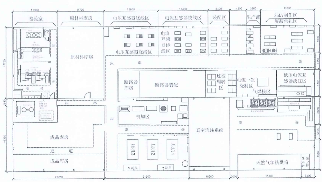
厂区布局图
