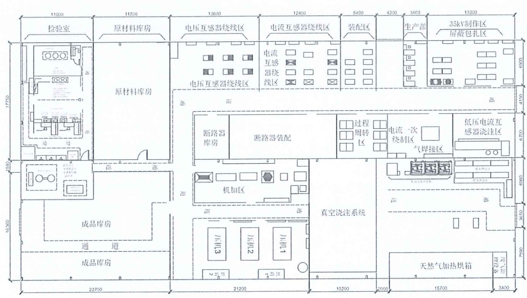
厂区布局图
