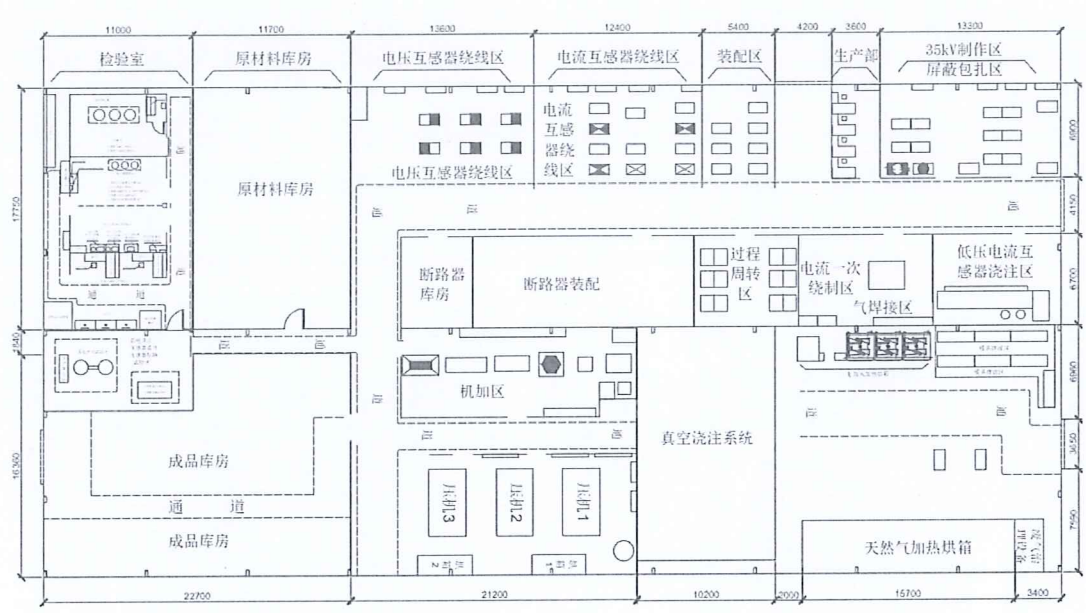
厂区布局图
