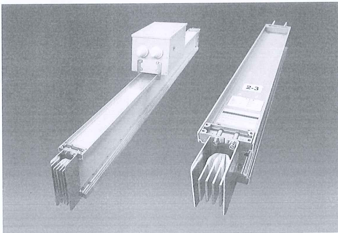
母线槽产品
