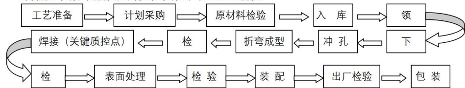
2.高低压母线、交流固定式机架母线生产加工工艺流程：
