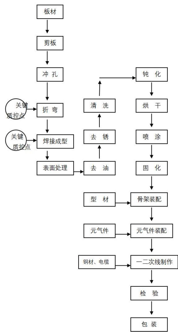
1. 高低压开关柜、箱，无功补偿柜，箱变生产加工工艺流程图：
