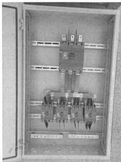
配电箱 PXT
