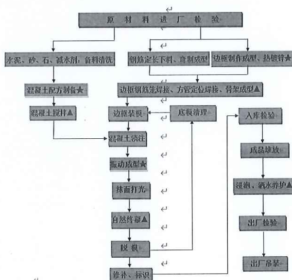
装配式混凝土盖板生产工艺流程图
