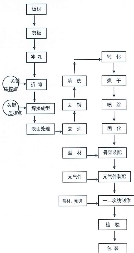
1. 高低压开关柜、箱，无功补偿柜，箱变生产加工工艺流程图：
