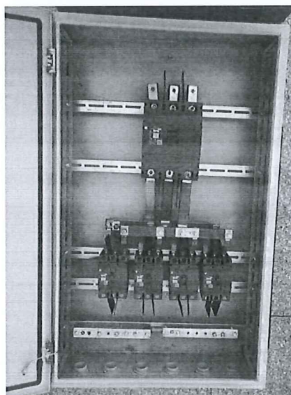
配电箱 PXT
