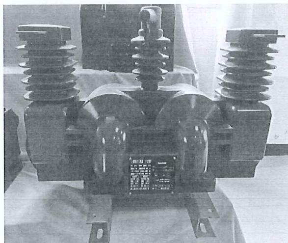
组合互感器
