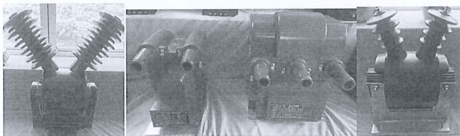
组合互感器
