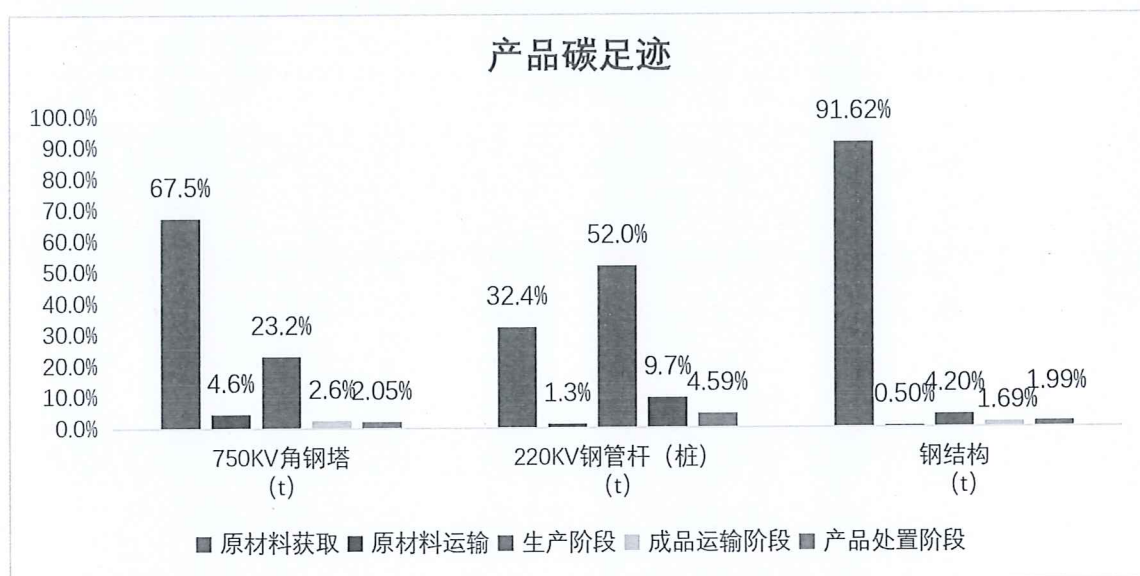
图 5.2.2-1 生命周期阶段碳排放分布图
