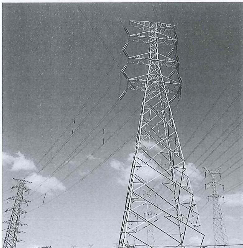
750KV 角钢塔
