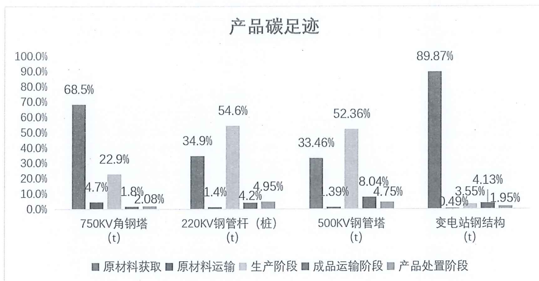
图 5.2.2-1 生命周期阶段碳排放分布图
