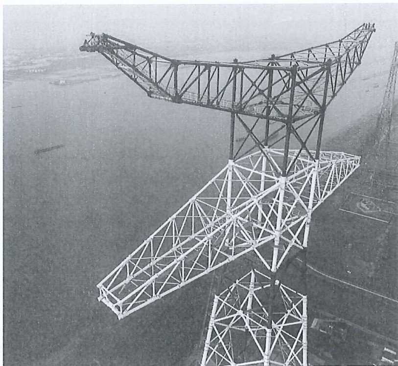
500KV 钢管塔
