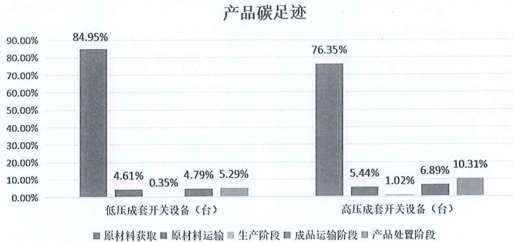
图 5.2-3 生命周期阶段碳排放分布图
