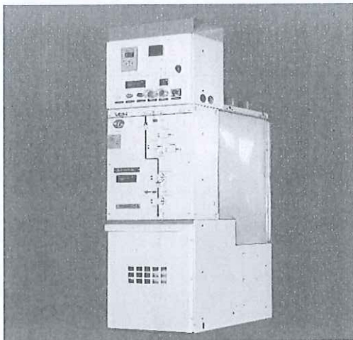
环网柜
