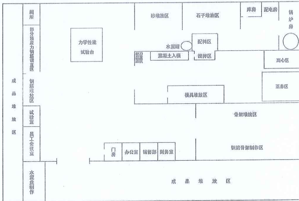
厂区布局图
