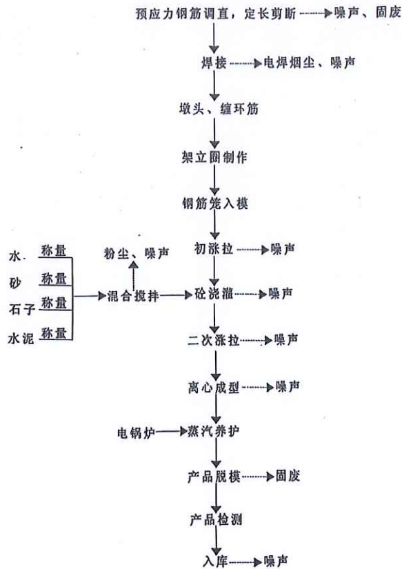
工艺流程图：
