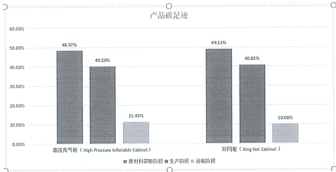
图 5.2-3 生命周期阶段碳排放分布图
